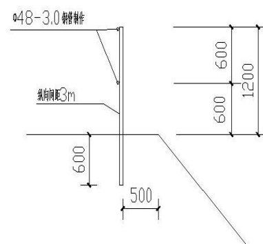
基坑顶栏杆大样
