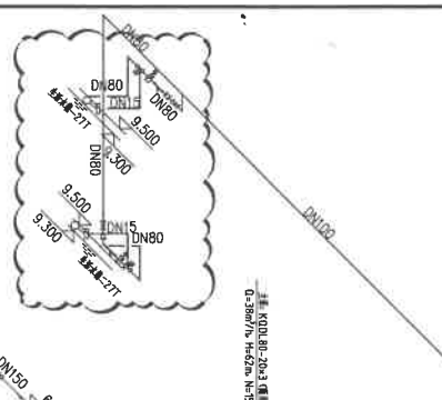
生活水箱供水管系统图
