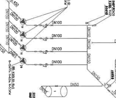
生活水箱进水管系统图
