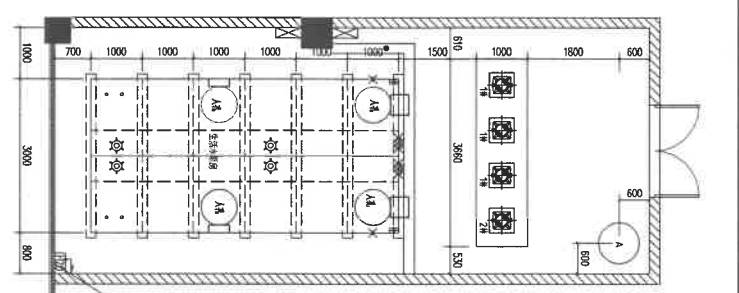
生活水泵房设备、基础定位图 150
